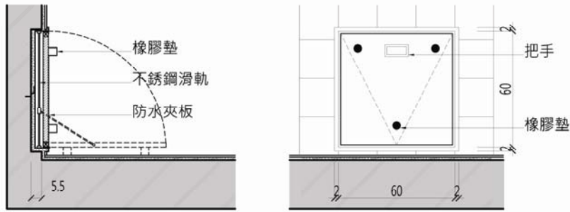
圖 3-20 換裝平台之使用與收納狀態
