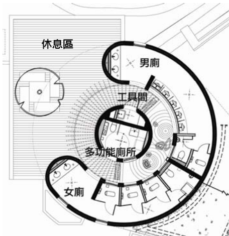
圖 2-5 庭園式之戶外景觀等待空間案例(塔塔加公廁)
