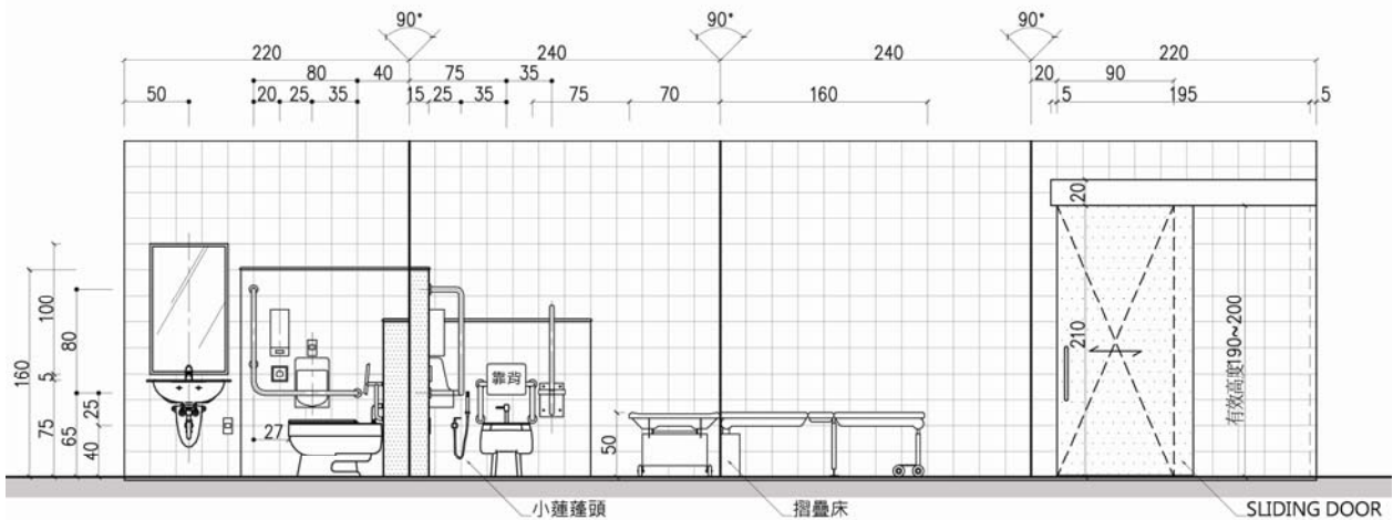
圖 3-49 行動不便廁所 A 型-設計展開立面圖
