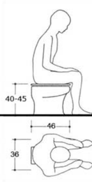
圖 3-4 成人用坐式便器參圖
