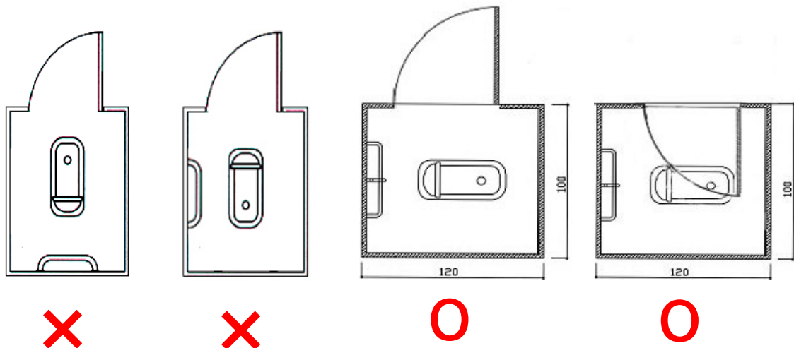
圖 3-6 蹲式便器設置方向應與門平行
