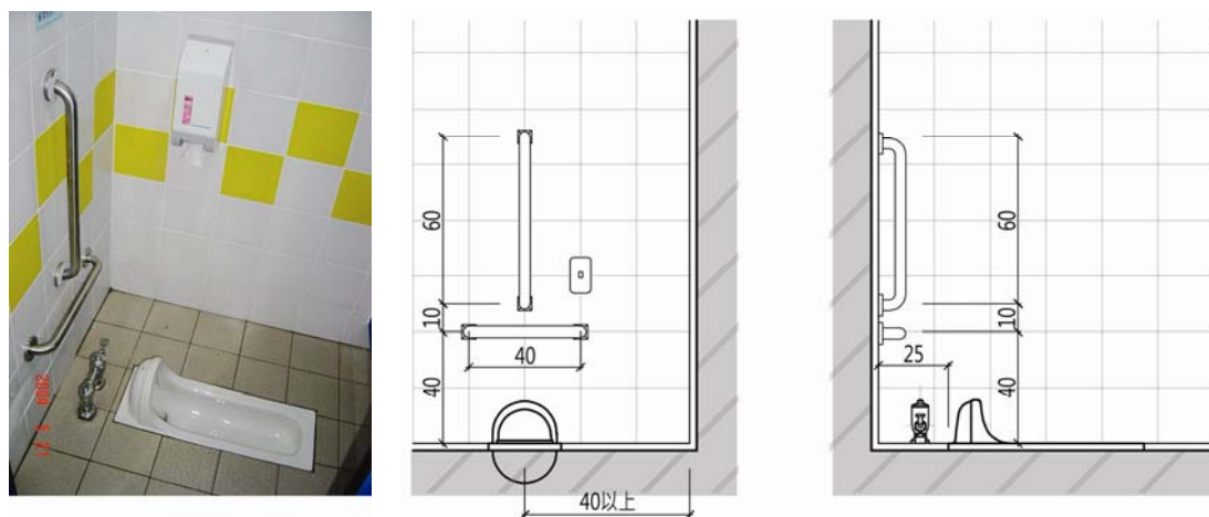
圖 3-11 輔助蹲下站立之扶手
