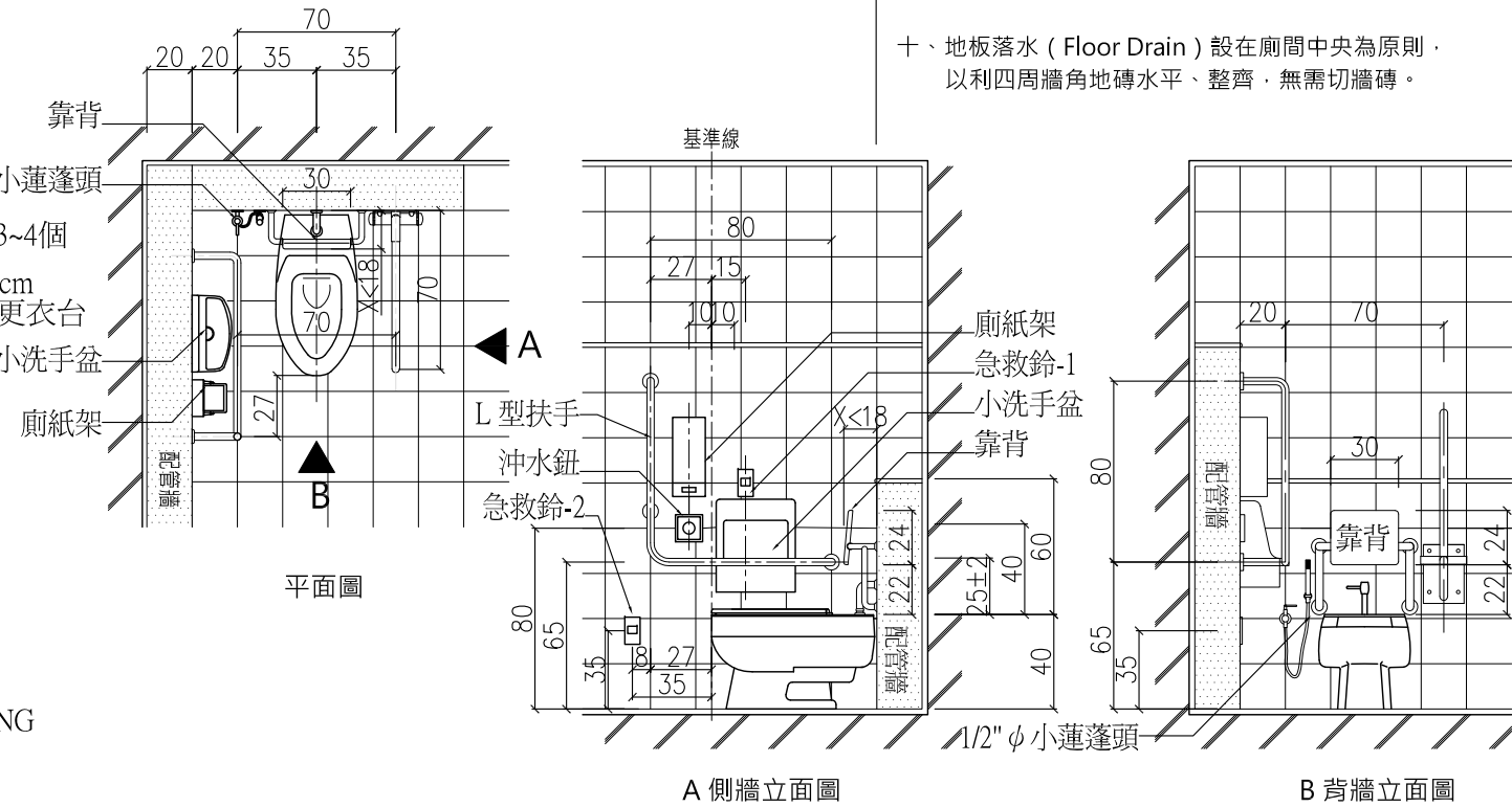
行動不便者廁所-馬桶周圍設備標準圖
