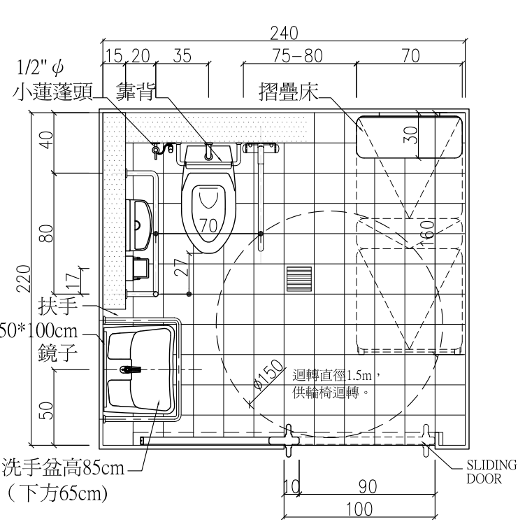
A-PLAN 行動不便者廁所內 加裝摺疊床，可供脊椎受傷患者使用
