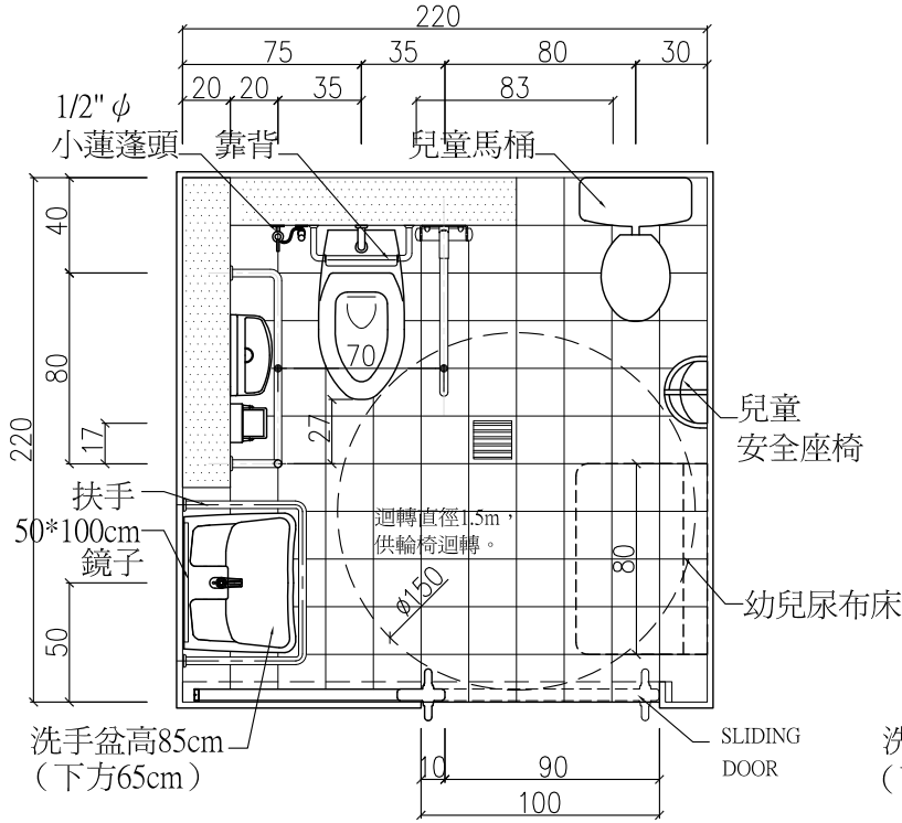
B-PLAN 行動不便者廁所內加設親子廁所
