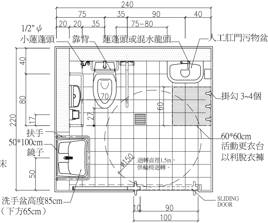
C-PLAN 行動不便者廁所內加人工肛門廁所
