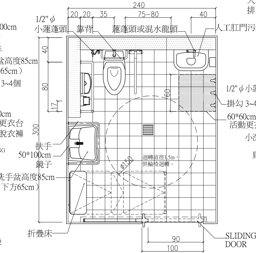
E-PLAN 多功能行動不便者廁所
